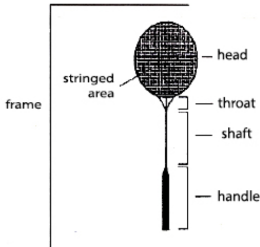
Gambar 3.8 Bagian Utama Raket
